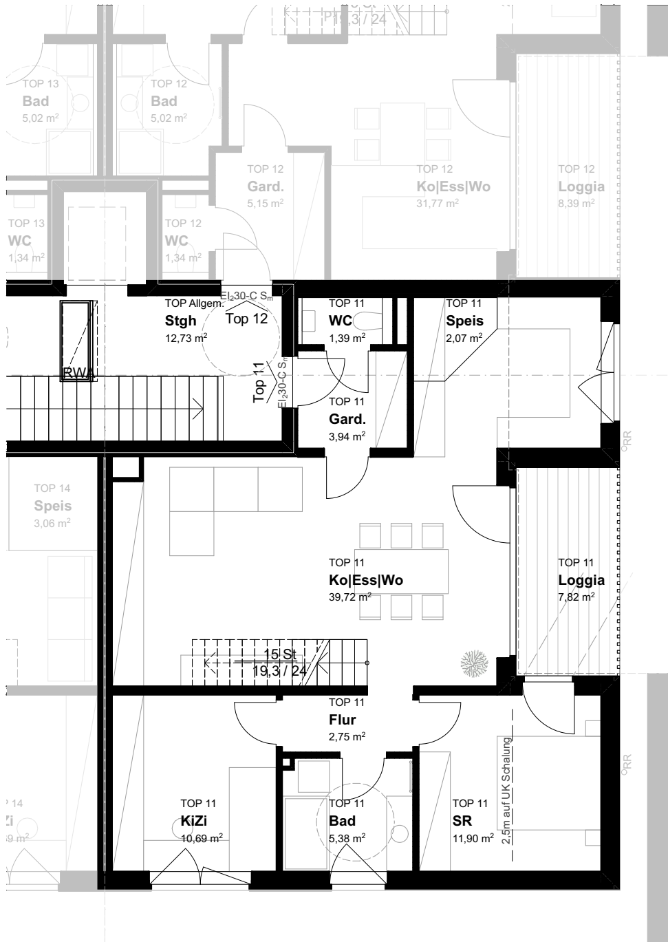
3. OBERGESCHOSS
