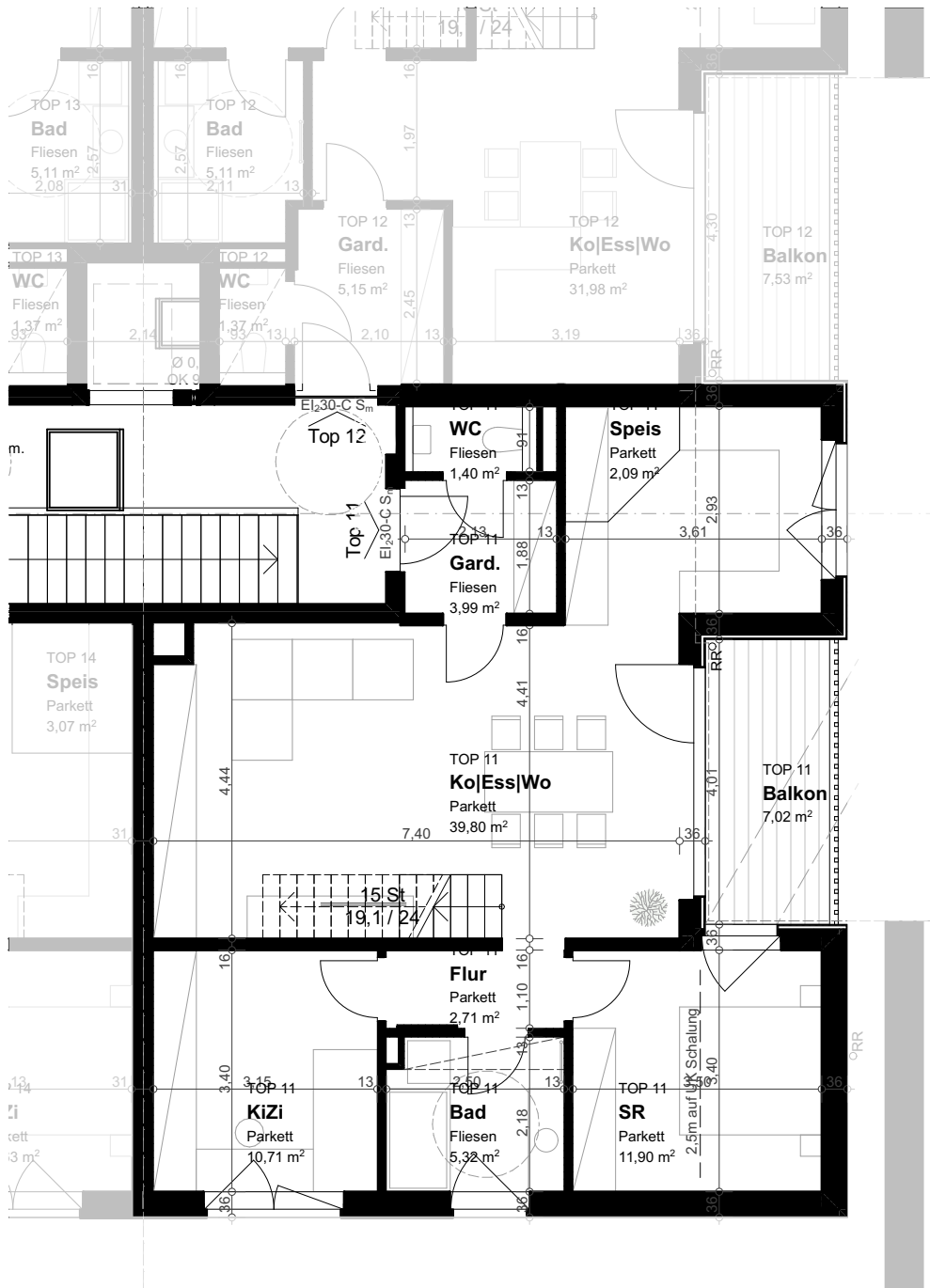
3. OBERGESCHOSS
