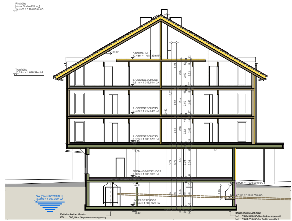
Schnitt A-A
