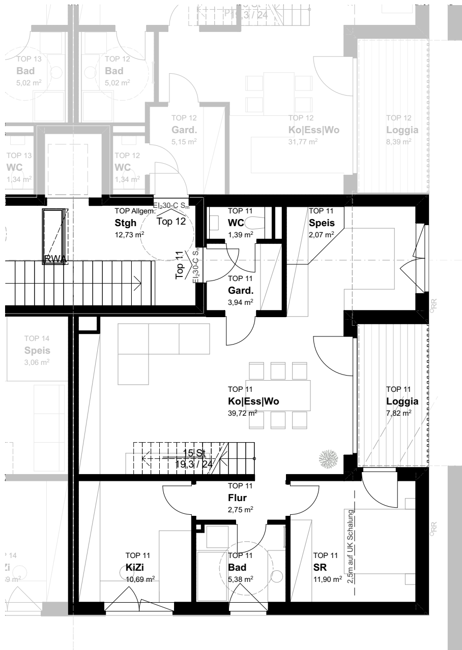
3. OBERGESCHOSS
