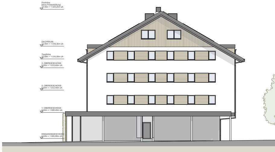
ANSICHT NORD
