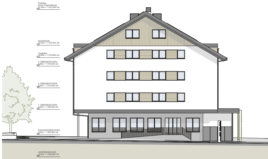
ANSICHT SÜD
